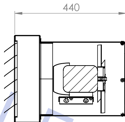
SEÇÃO A-A ESCALA 1 : 9
