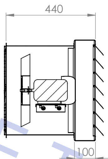
SEÇÃO A-A ESCALA 1 : 12
