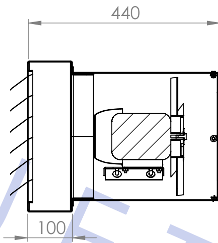
SEÇÃO A-A ESCALA 1:9
