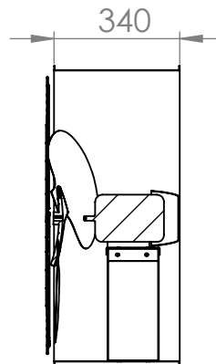
SEÇÃO A-A ESCALA 1:19
